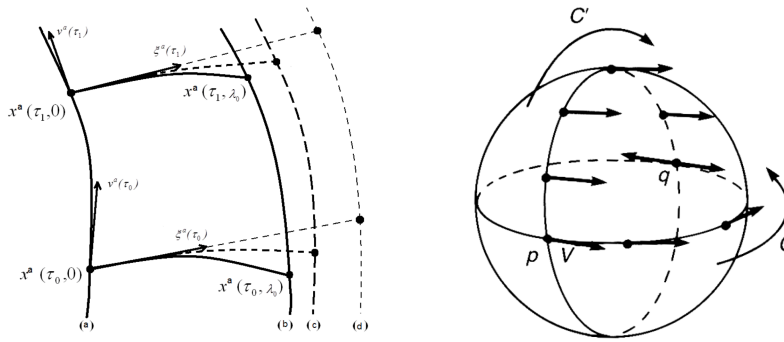
Figura 2: Derecha: transporte paralelo de p \rightarrow q , a lo largo de curvas C y C' , del vector \mathbf{V} . La figura muestra que, debido a la curvatura de la esfera, el vector obtenido en q depende del camino.
